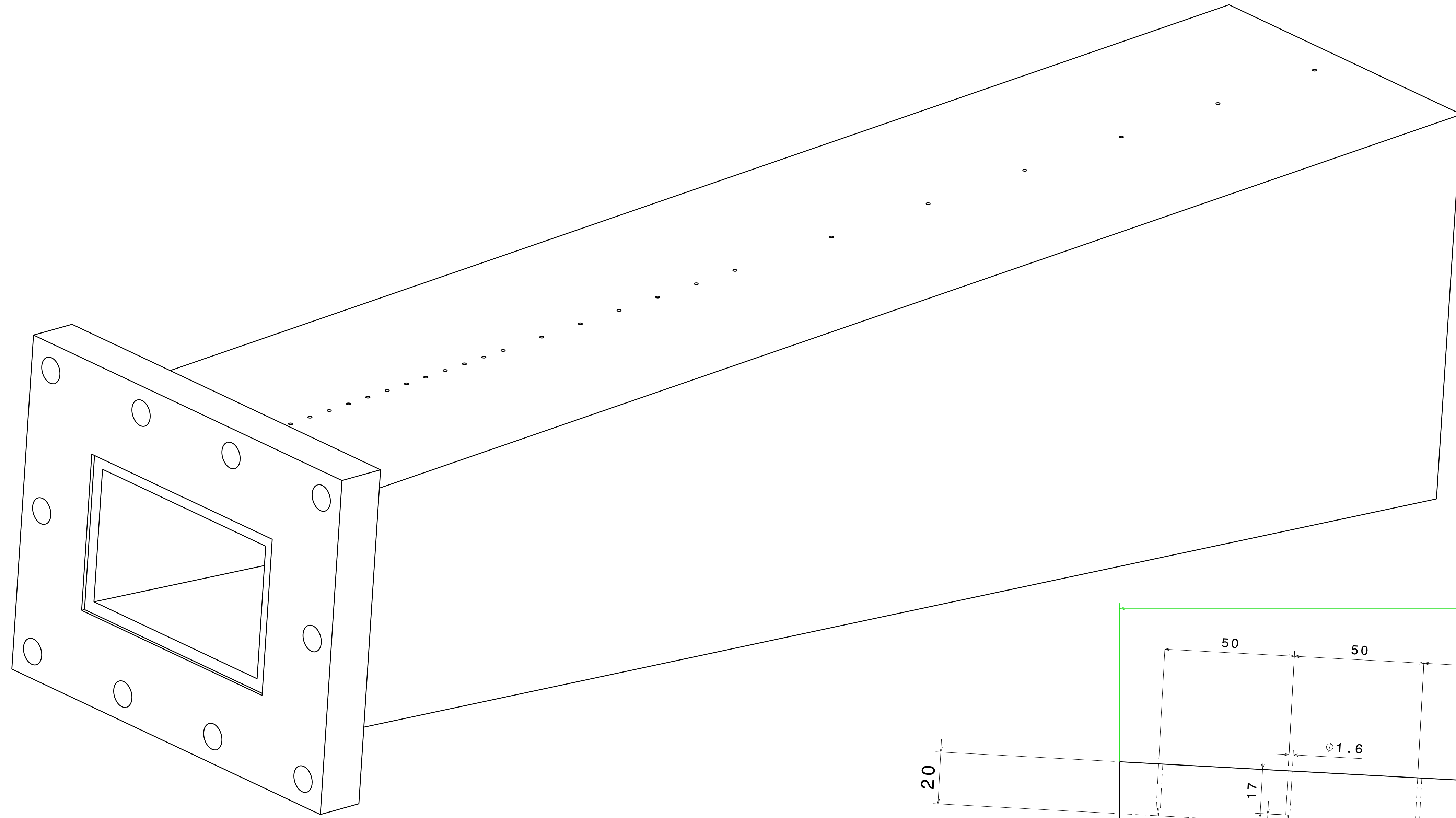
Isometric view Scale: 1:1
